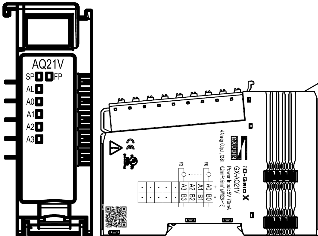
圖 4.25 GX-AQ21V 圖面
