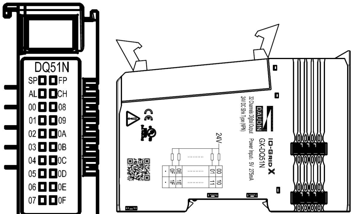
圖 4.15 GX-DQ51N 圖面
