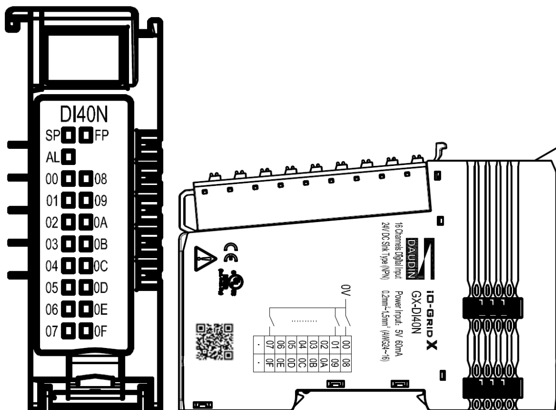
圖 4.4 GX-DI40N 圖面
