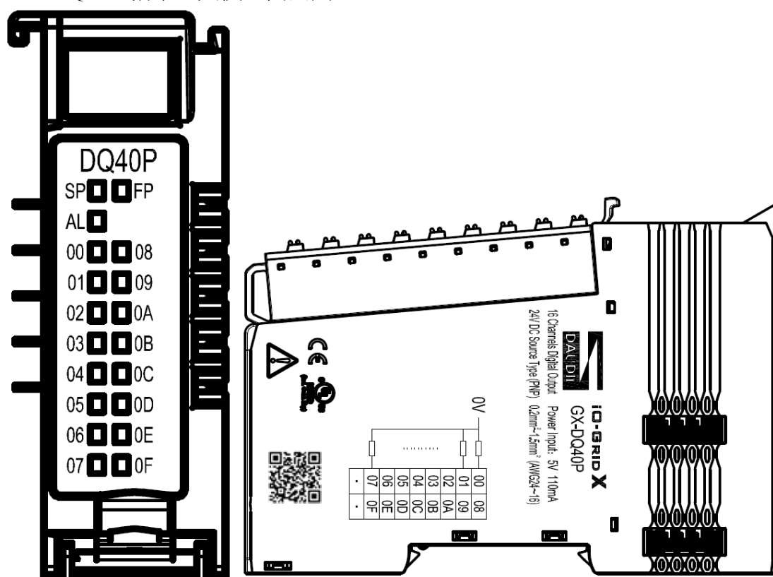
圖 4.12 GX-DQ40P 圖面
