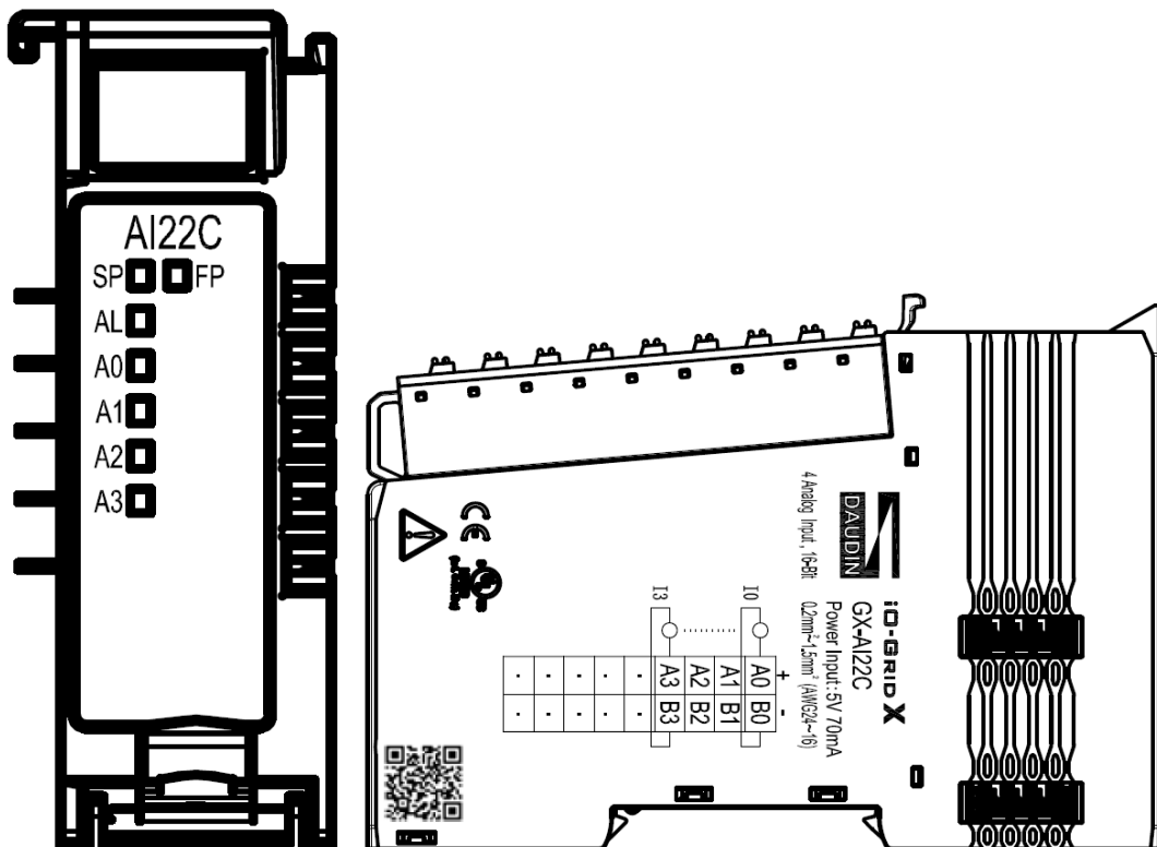
圖 4. 20 GX-AI22C 圖面
