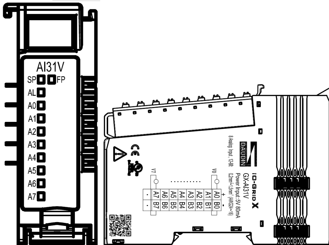
圖 4.21 GX-AI31V 圖面
