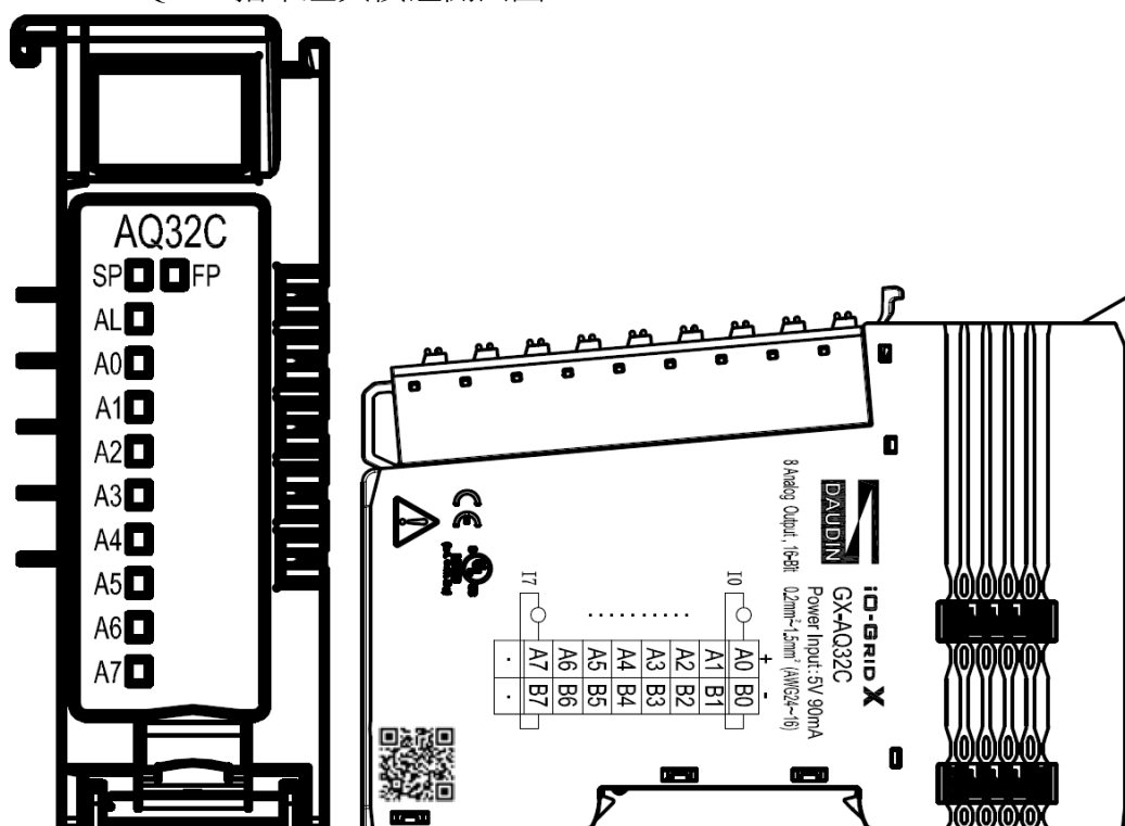
圖 4. 32 GX-AQ32C 圖面
