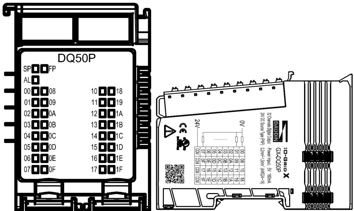
圖 4.14 GX-DQ50P 圖面
