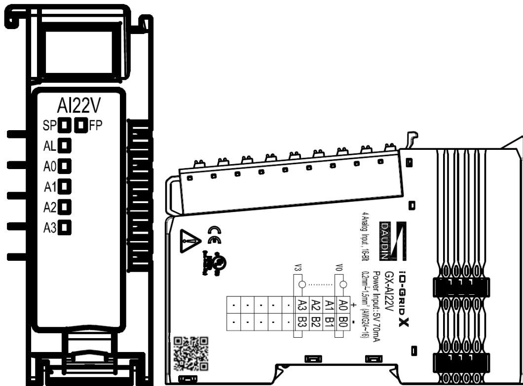
圖 4. 19 GX-AI22V 圖面
