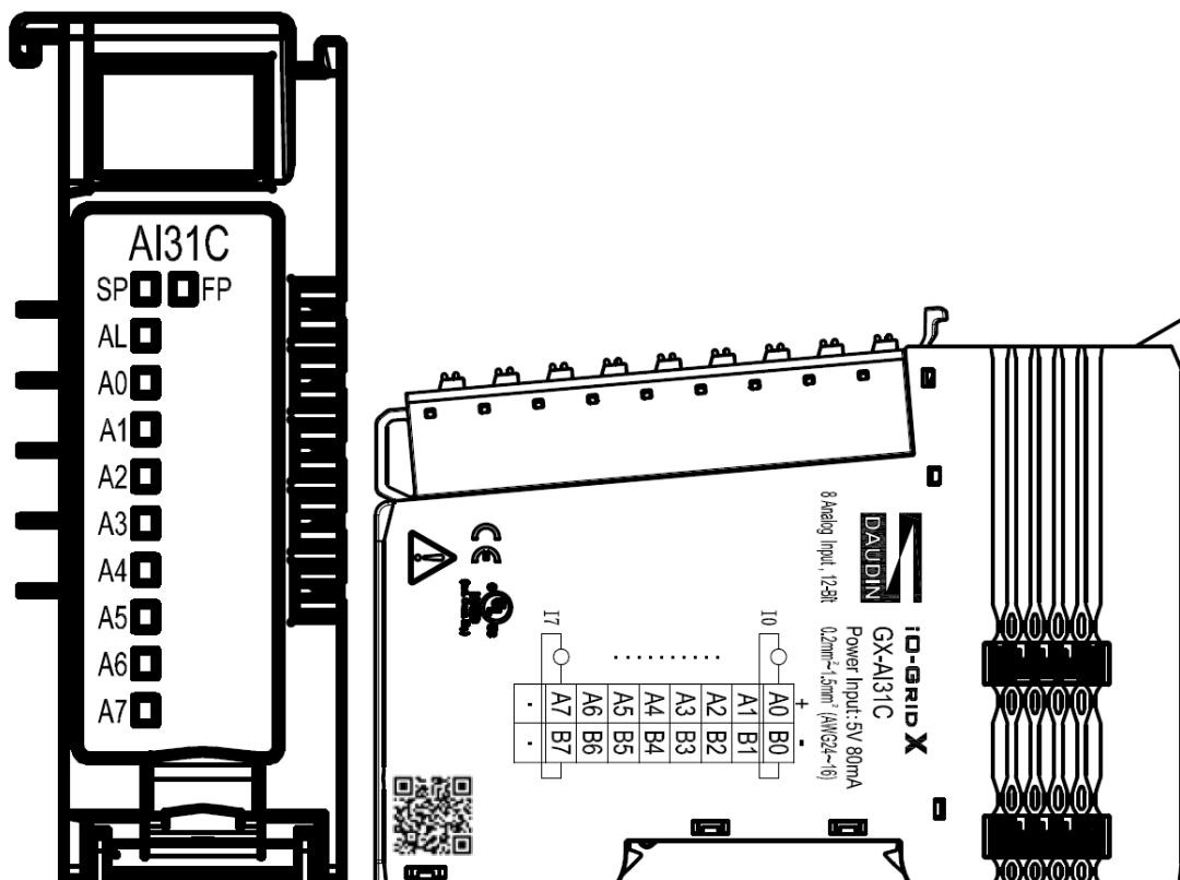
圖 4.22 GX-AI31C 圖面
