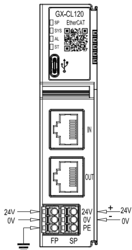
圖 8.1 耦合器接線圖
