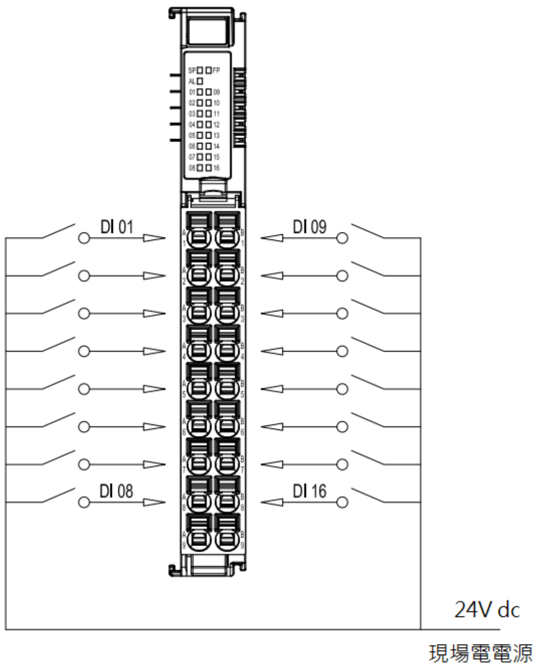
圖 8.3 GX-DI40P 接線圖
